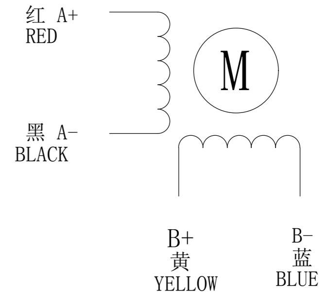
接线图/WIRING DIAGRAM
